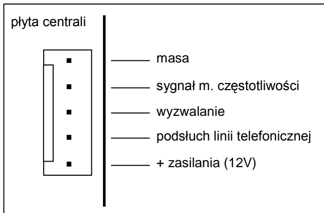
Rysunek 13. Gniazdo do podłączenia syntezera mowy SM-2
