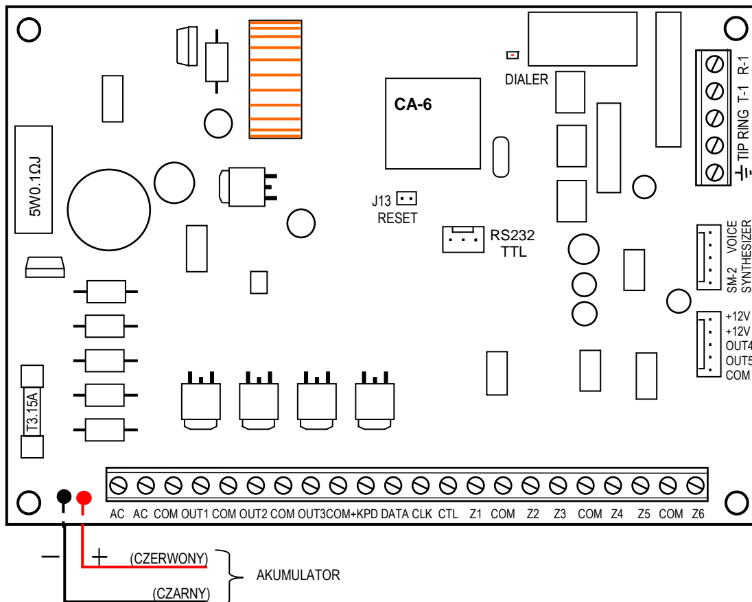
Rysunek 2. - Widok schematyczny płyty głównej centrali CA-6 wykonanej w wersji CA6P V4.1.
