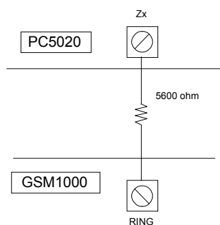
Rys. 15. Linia odpowiedzi modułu GSM.
