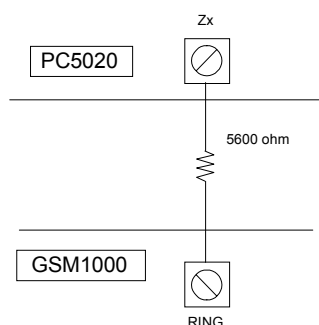
Rys. 15. Linia odpowiedzi modułu GSM.
