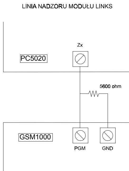
Rys. 14. Linia nadzorowania modułu GSM.
