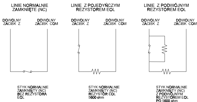
Rys. 13. Podłączenie linii do wyłączenia/włączenia systemu kluczem.
