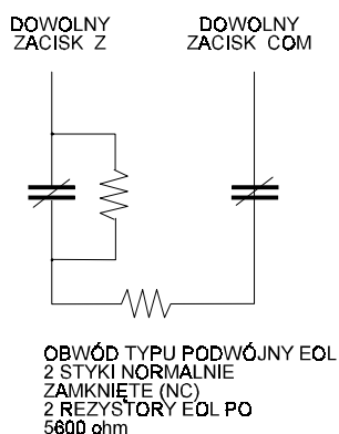
Rys. 10. Linia dozorowa z podwójnym rezystorem końcowym (DEOL).
