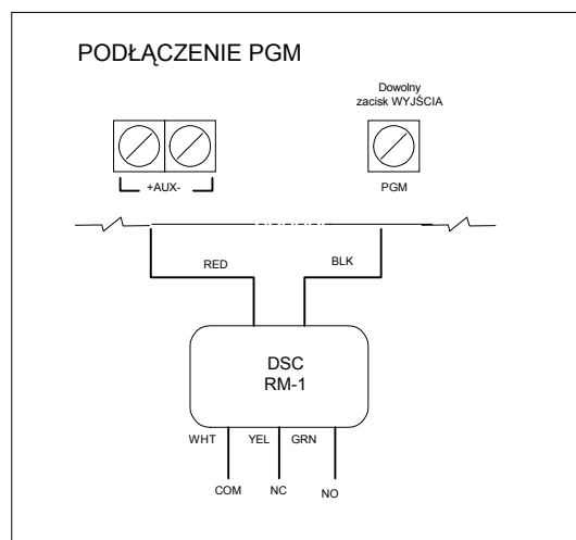
Rys. 3. Podłączenie wyjść PGM
