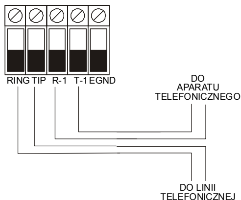
Rys. 4. Podłączenie linii telefonicznej
