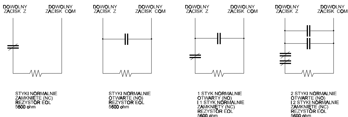
Rys. 9. Linie dozorowe z pojedynczym rezystorem końcowym (EOL).
