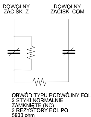
Rys. 10. Linia dozorowa z podwójnym rezystorem końcowym (DEOL).
